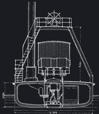
Querschnitt Trajectdampfer
